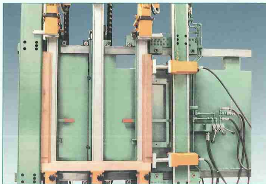
Größeneinstellung mit Einzelhölzern und losem Ein- legen in die Presse Euronova Z
