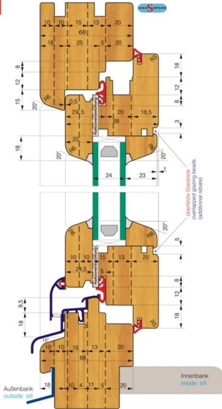
Konstruktionsdetail: Vertikalschnitt construction detail: vertical section
